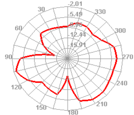
820.000MHz H
