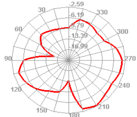
820.000MHz E2
