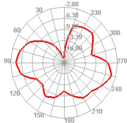
670.000MHz E2
