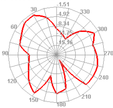
1740.000MHz E1
