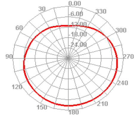
820.000MHz E2
