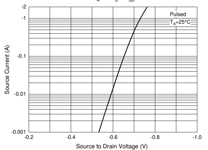
Fig. 6 - I_S - V_{SD}
