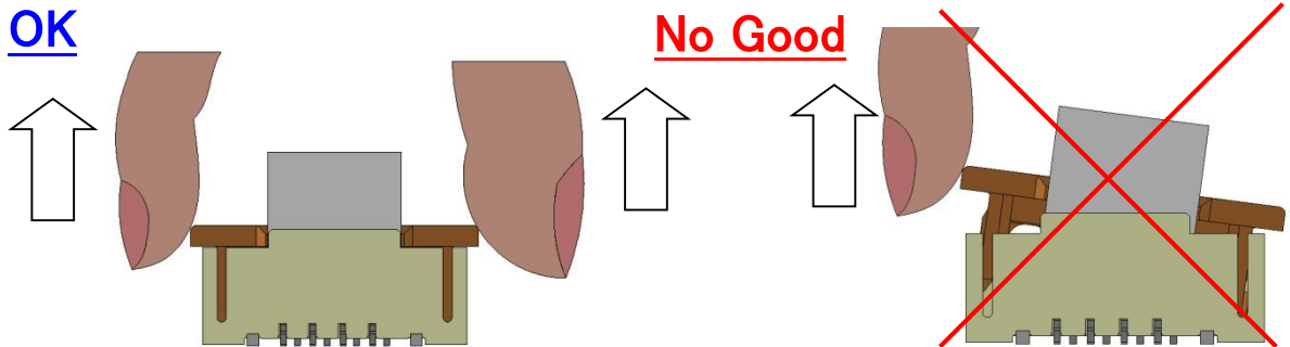
アクチュエータの両側での操作 Pushing on both sides of actuator
