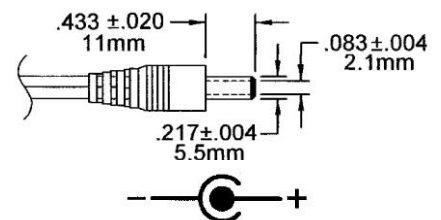
Dim.: mm
