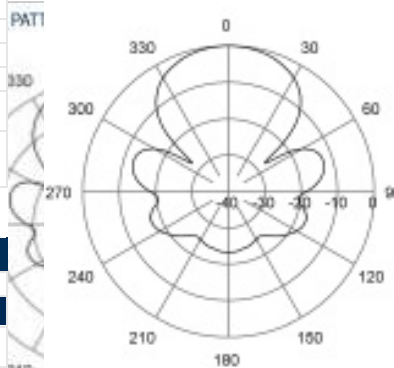
H-Plane | 155 MHz
