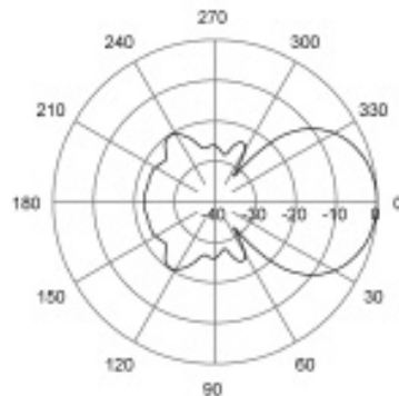
E-Plane | 155 MHz
