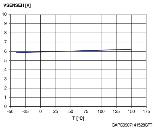
Figure 29: Vsenseh vs. Tcase
