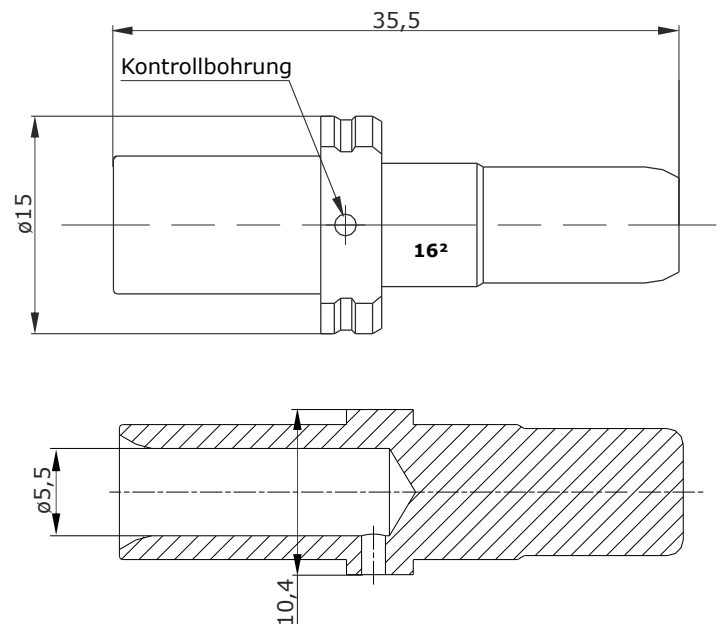
Hauptabmessungen Kontaktstift
