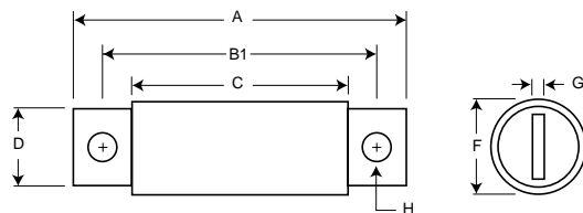
Fig. 1: 1-30 & 450-1000 Amp Range
