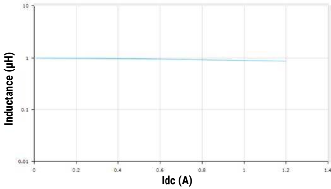
L1008Q1R0MDMIT
