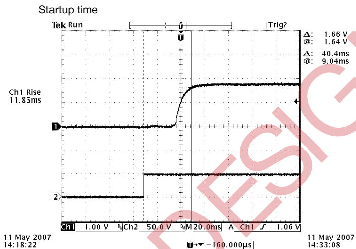
CH1: Vout
