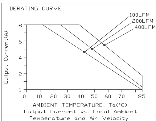
xRSB-40U05x, Vin=24V
