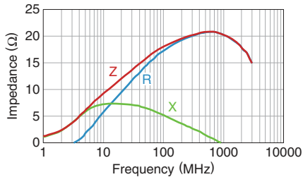
MMZ2012R150AT000
