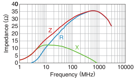
MMZ2012R300AT000
