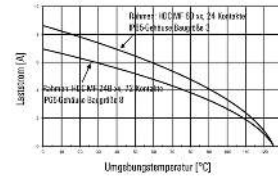
HDC-MHD 12-Module im IP65-Gehäuse, Leiter HD7V-K2,5:
