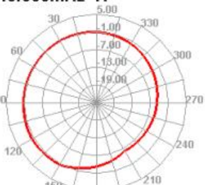
840.000MHz H
