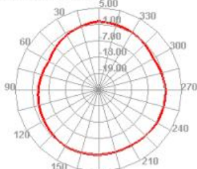
2200.000MHz H
