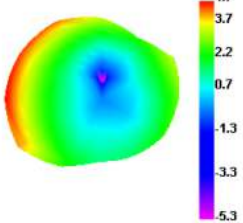
2650.000MHz E1
