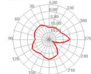
1000.000MHz E2
