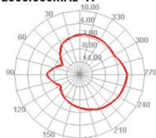
2500.000MHz E2
