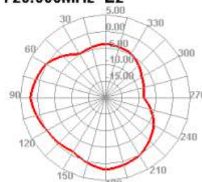
720.000MHz E2
