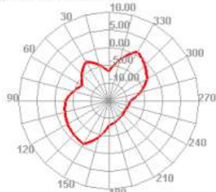
2400.000MHz E1
