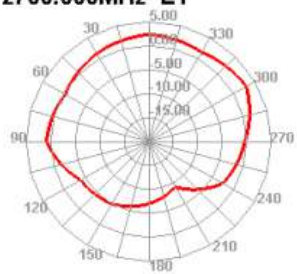
2700.000MHz E1
