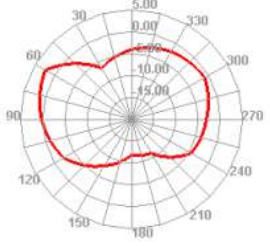
2650.000MHz E2
