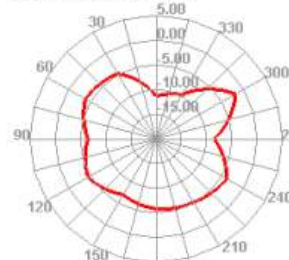
1000.000MHz E1
