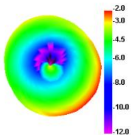
1560.000MHz E1
