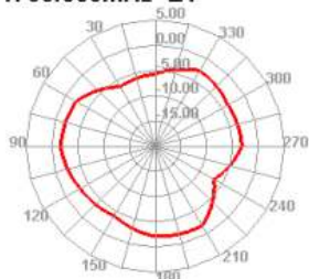
1700.000MHz E1
