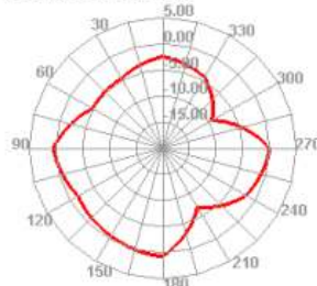
700.000MHz E1
