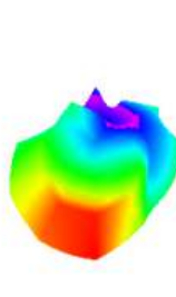
2450.000MHz E1
