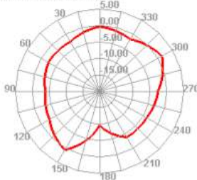
2500.000MHz E1
