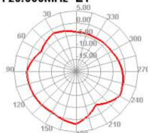
720.000MHz E1
