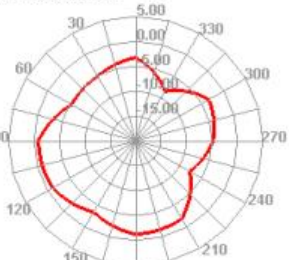
840.000MHz E2
