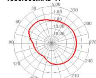
1000.000MHz H
