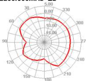
2200.000MHz E2
