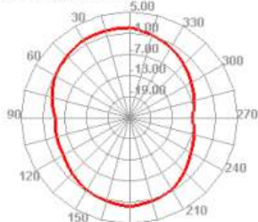
700.000MHz E2
