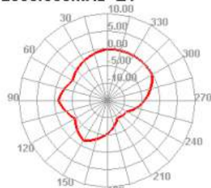
2500.000MHz E1
