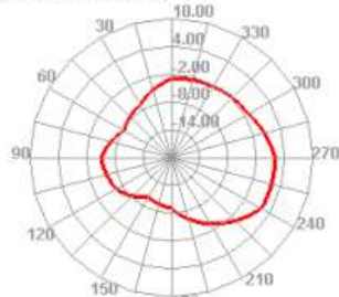
2400.000MHz E2
