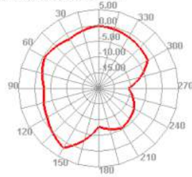
2450.000MHz E1
