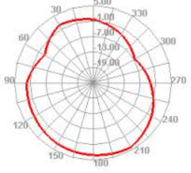
2650.000MHz E2
