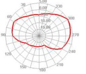
2650.000MHz E1
