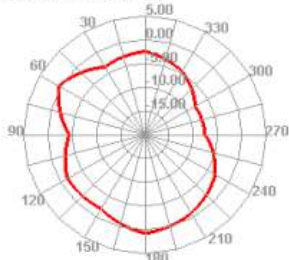
700.000MHz E2
