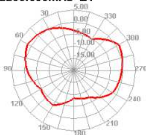
2200.000MHz E1
