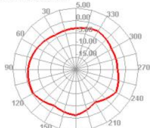
840.000MHz E1
