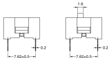
Flat Actuator
