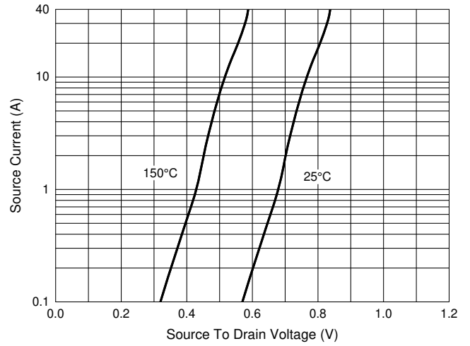
Fig. 2 - I S —V SD
