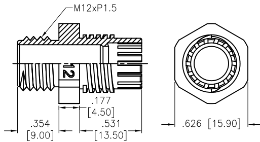
Ⓒ Body
