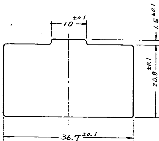
パネル取付穴寸法
