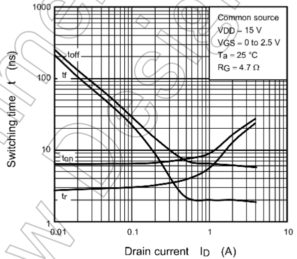
Fig. 7.10 t - I_D
