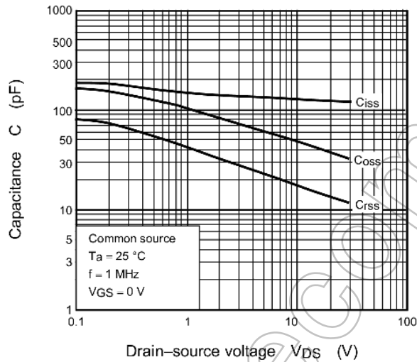
Fig. 7.9 C - V_{DS}
