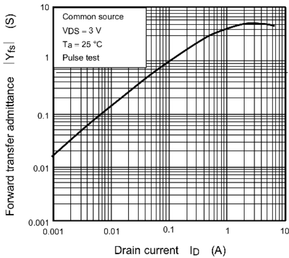
Fig. 7.7 |Y_{fs}| - I_D
