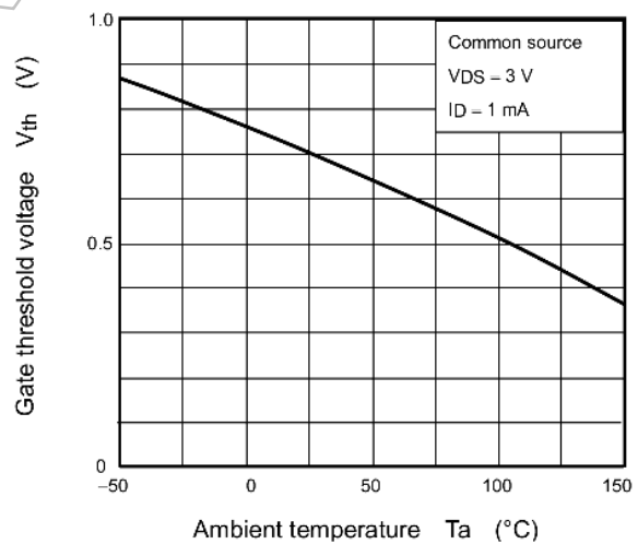
Fig. 7.6 Vth - Ta
