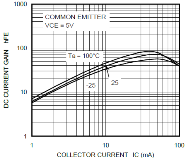
Fig. 10.14 RN1317 h_{FE}-I_c
