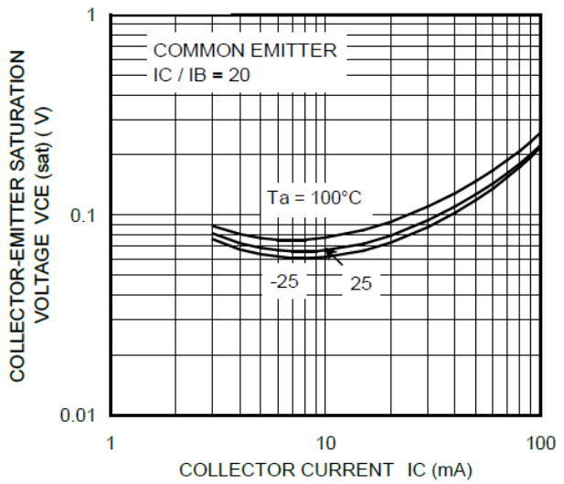
Fig. 10.16 RN1314 V_{CE(sat)}-I_c
