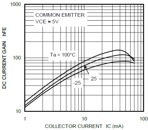
Fig. 10.15 RN1318 h_{FE}-I_c
