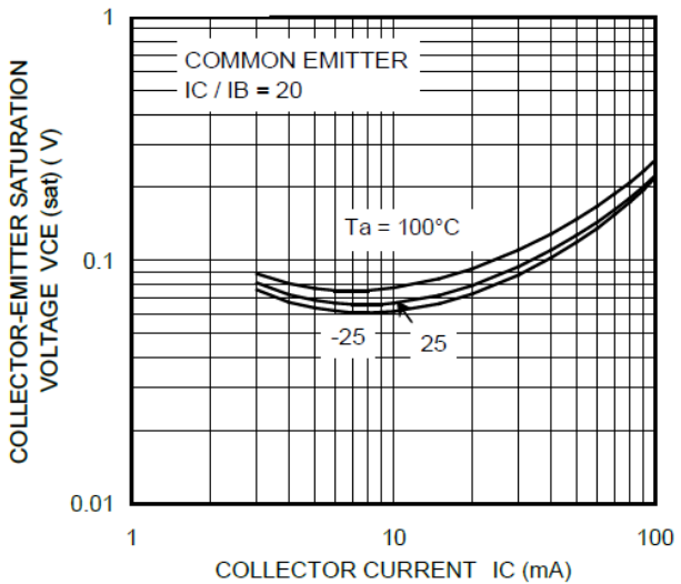
Fig. 10.17 RN1315 V_{CE(sat)}-I_c
