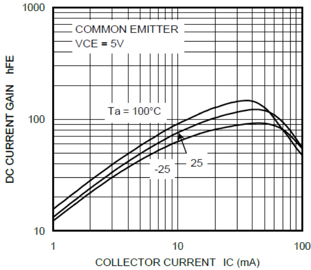
Fig. 10.13 RN1316 h_{FE}-I_c
