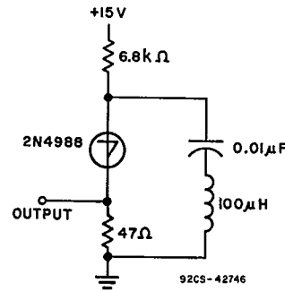
Fig. 20—10 kHz oscillator circuit.
