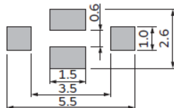
NFM41CC/41PC
