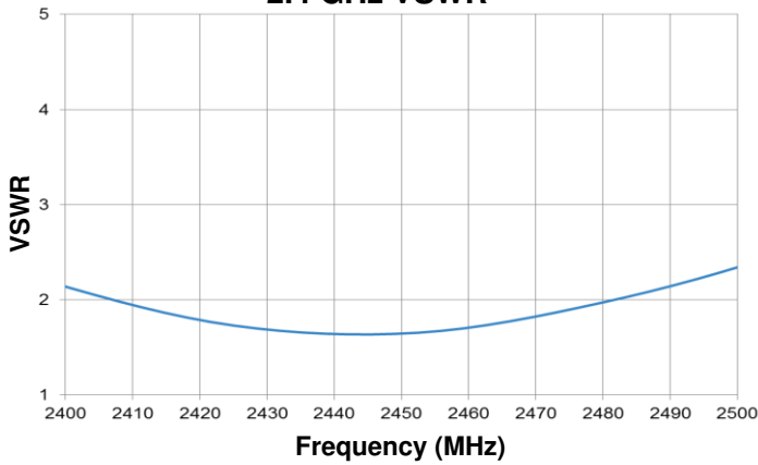
2.4 GHz VSWR
