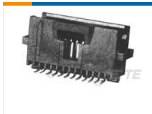
TE Part #5-147377-1 10 SYS50 SMT HDR DR SHD SN
