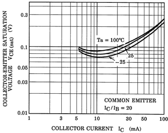
Fig. 10.19 RN1101 V_{CE(sat)} - I_C
