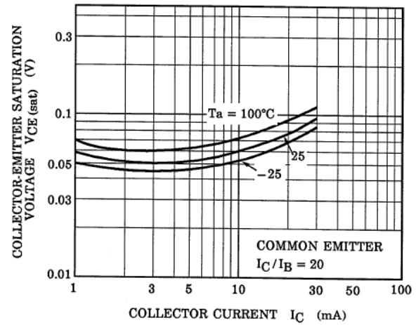
Fig. 10.22 RN1104 V_{CE(sat)} - I_C
