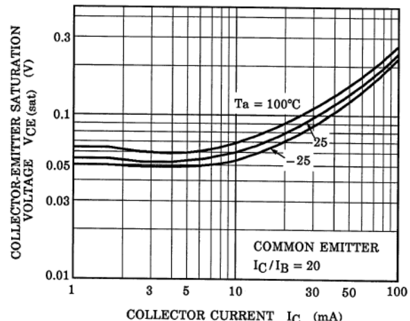
Fig. 10.24 RN1106 V_{CE(sat)} - I_C
