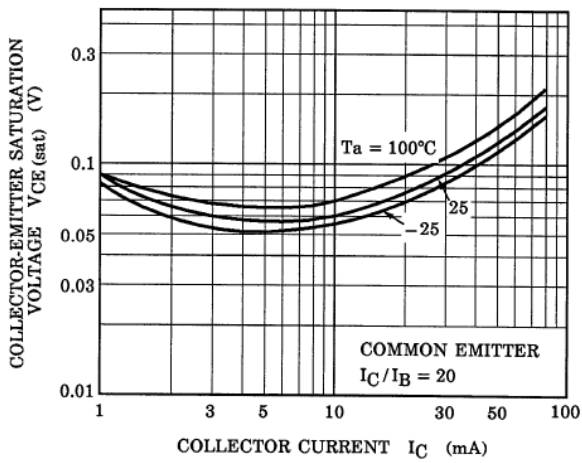
Fig. 10.21 RN1103 V_{CE(sat)} - I_C
