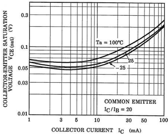
Fig. 10.23 RN1105 V_{CE(sat)} - I_C
