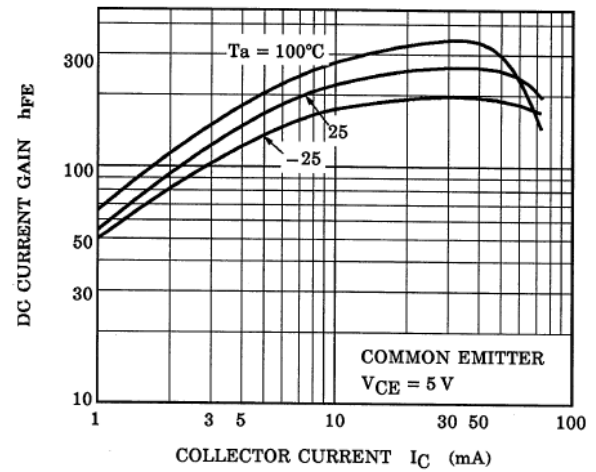
Fig. 10.16 RN1104 h_{FE}-I_C
