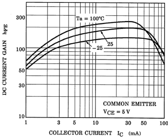
Fig. 10.17 RN1105 h_{FE}-I_C
