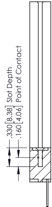
SECTION A-A
