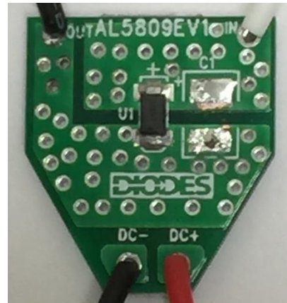
AL5809EV1 (PDI123)
