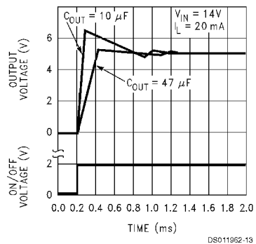
Enable Transient
