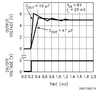
Enable Transient
