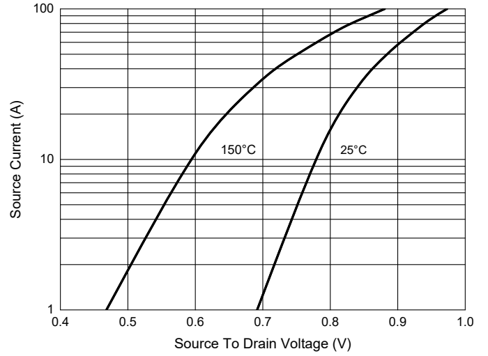
Fig. 2 - I_s - V_{SD}
