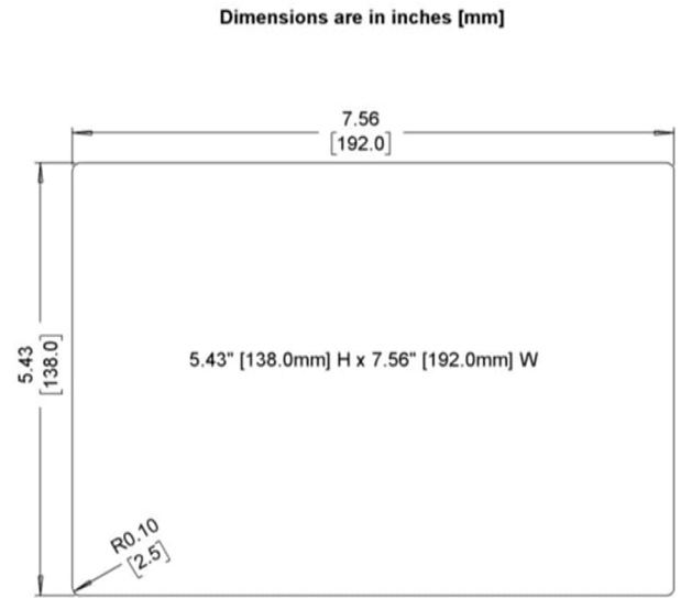
Cutout Dimensions
