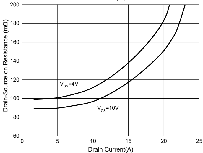
Fig. 5 - R_{DS(ON)} - I_D
