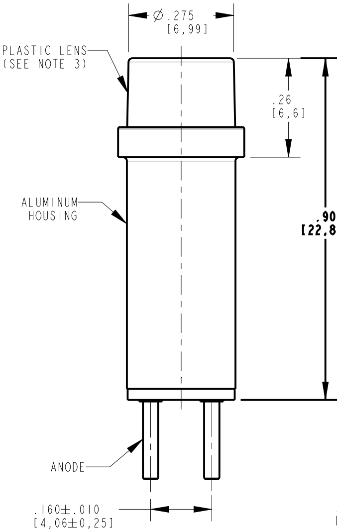
FIG. 1 (CYLINDRICAL LENS)
