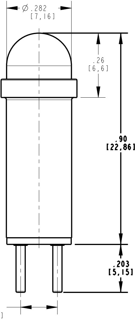
FIG. 2 (STOVEPIPE LENS)
