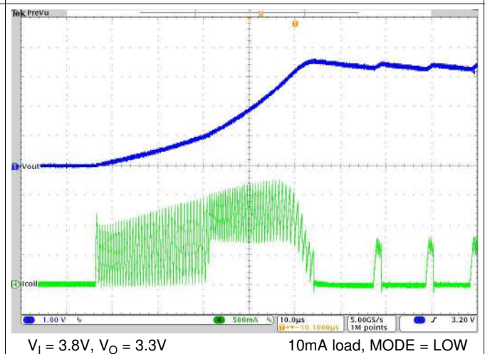
Figure 25. Softstart Waveforms in PFM Mode
