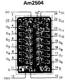
DIE SIZE 0.087" X 0.135"
