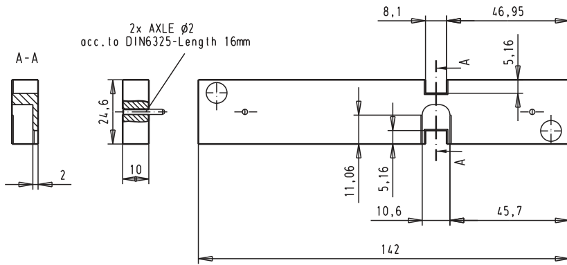
Part 2: har.mik LEFT GUIDE
