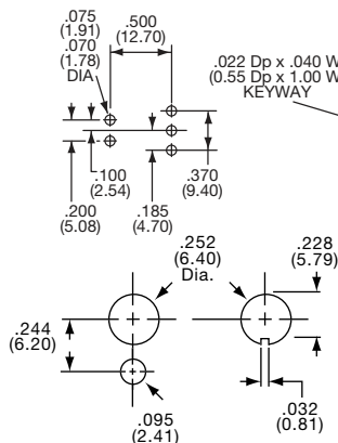
Horizontal Actuation
