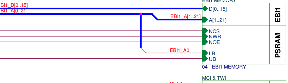
04 - EBI1 MEMORY
