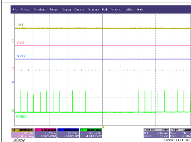
VIN = 0 V
