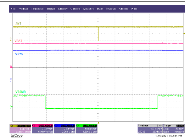
VIN = 5 V
