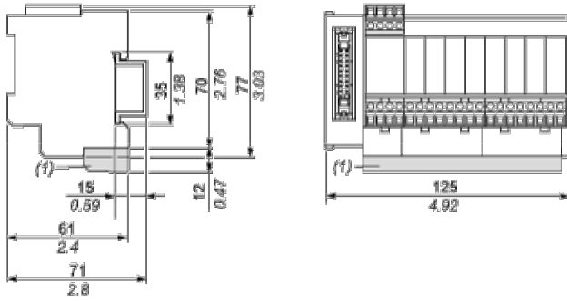
(1) ABE7BV10 / ABE7BV10E
