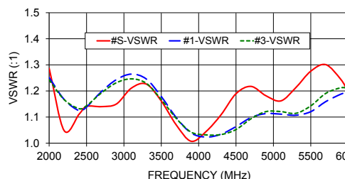
ZN4PD1-63-S+ VSWR
