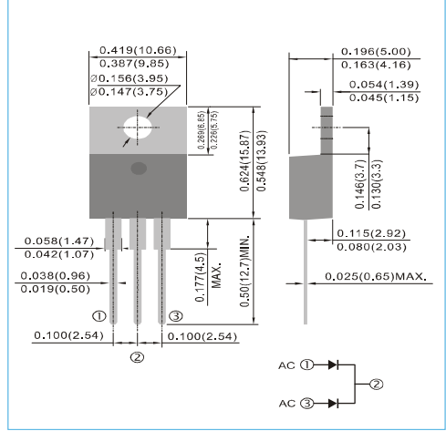
TO-220AB Unit : inch(mm)
