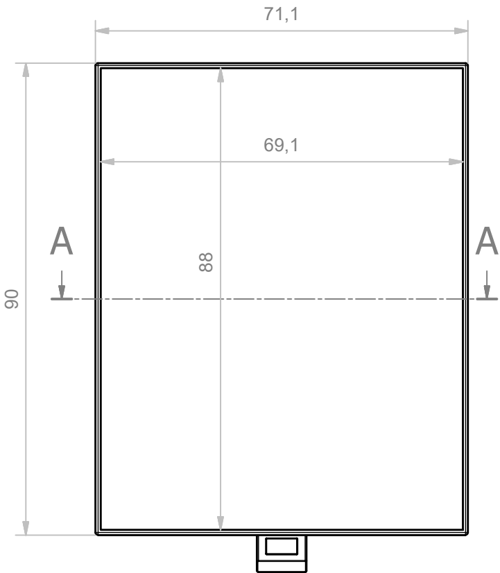
A-A (1:1)
