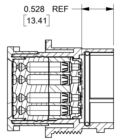
SECTION AA-AA
