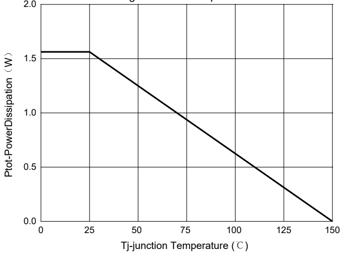
Fig. 11 - PowerDissipation
