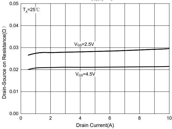
Fig. 9 - R_{DS(ON)} - I_D
