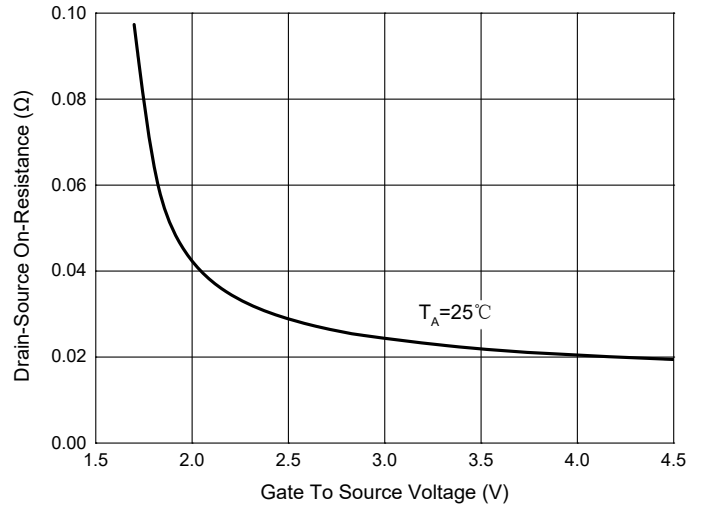
Fig. 8 - R_{DS(ON)} - V_{GS}
