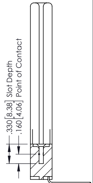
SECTION A-A
