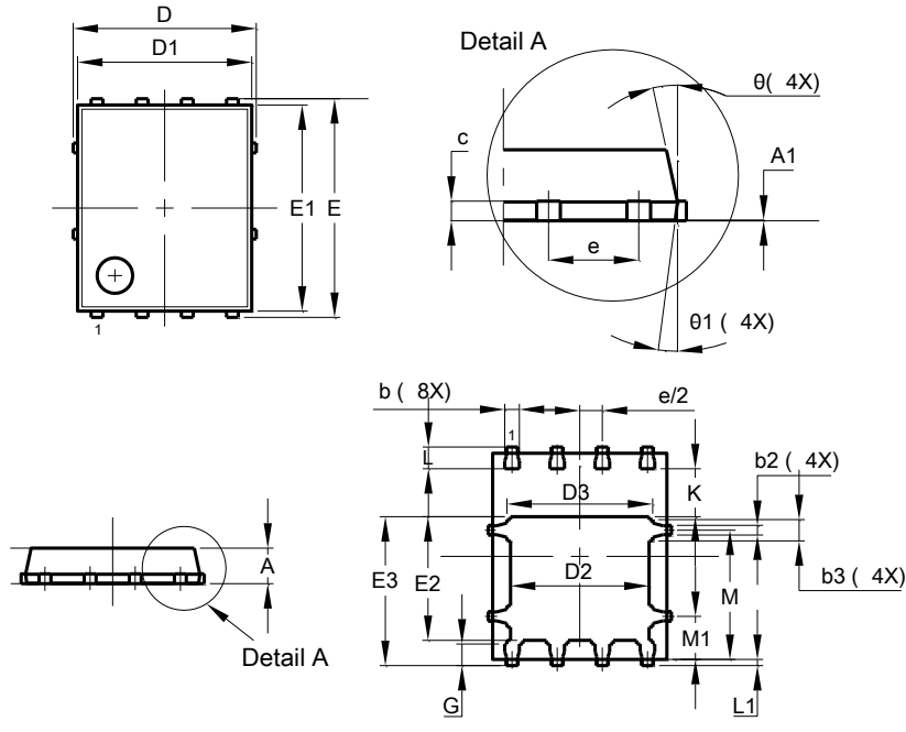
PowerDI5060-8
