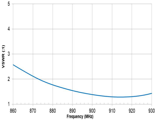
VSWR
