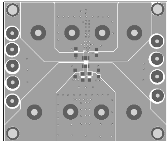
Figure 2—Top Layer
