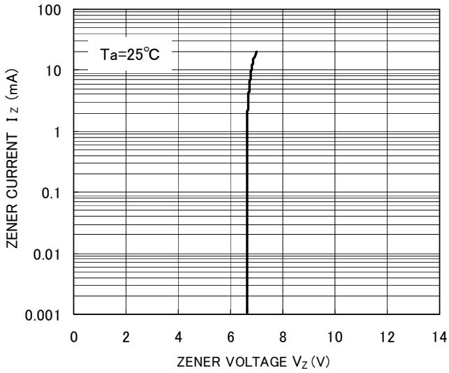
I_z - V_z
