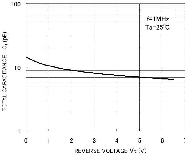
C_T - V_R
