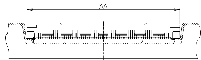
D-D (SCALE 2:1)
