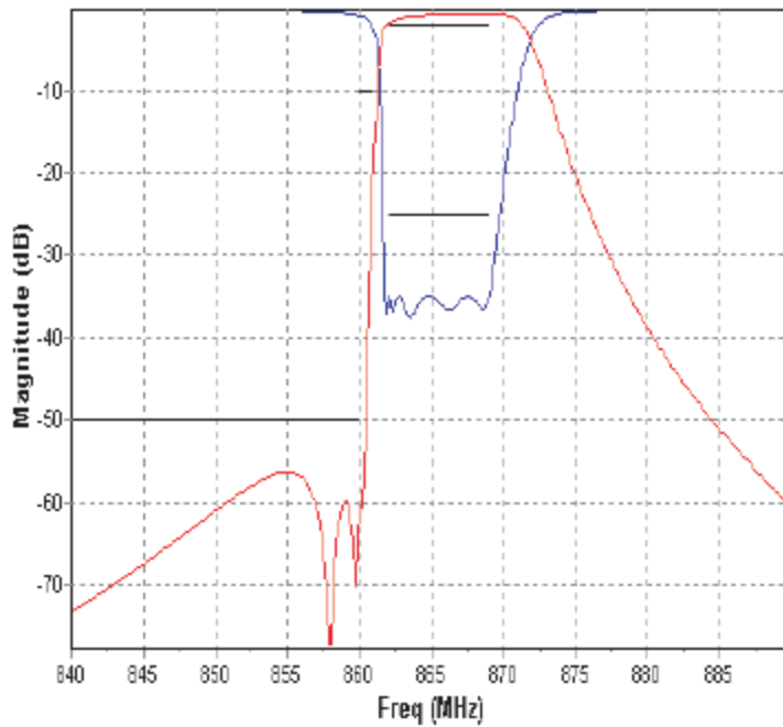
ANT-TX
